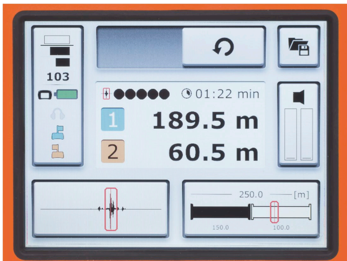
Resultado de medición en dos secciones de tuberías
